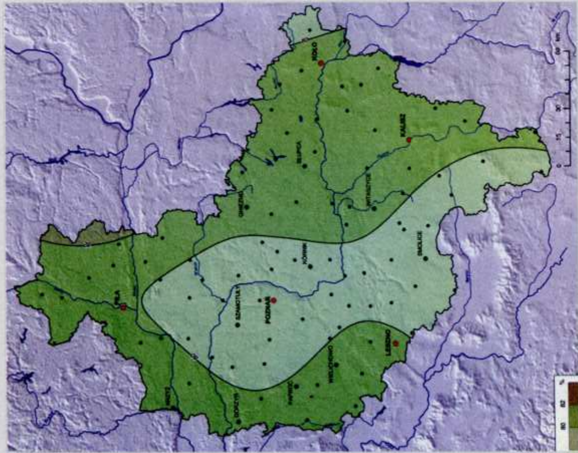
Mapka 5. Średnia roczna wilgotność względna powietrza (%)
