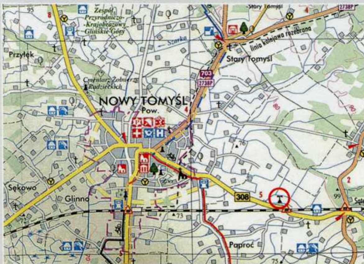
Mapka 1. Lokalizacja posterunku klimatologicznego w Paproci
