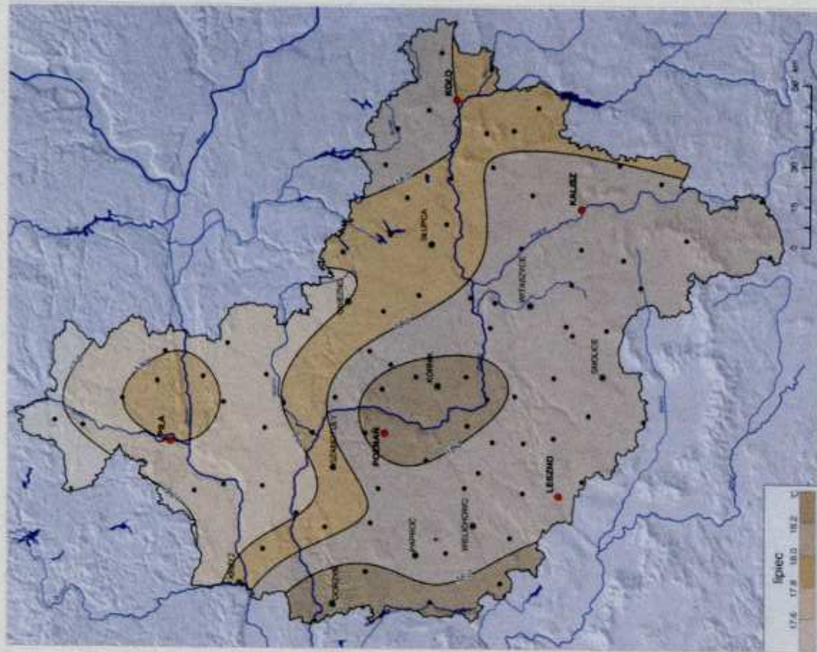
Mapka 4. Średnia temperatura powietrza - lipiec (C°)
