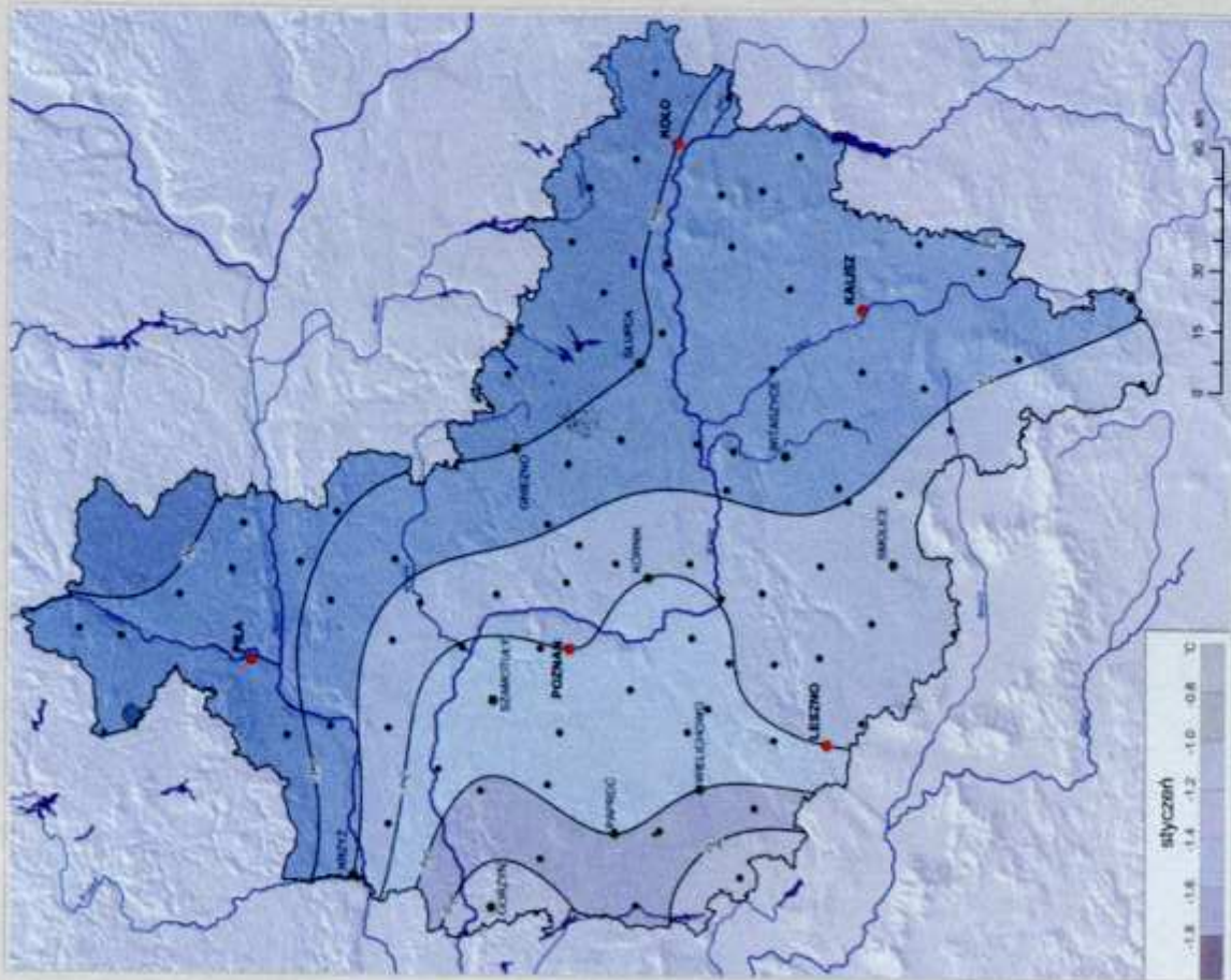
Mapka 3. Średnia temperatura powietrza - styczeń (C°)
